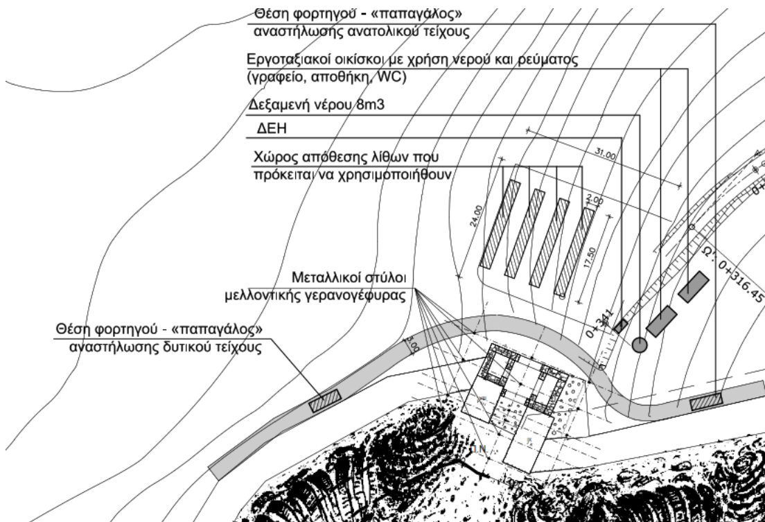
Εικόνα 2. Εργοταξιακός δρόμος κίνησης γερανοφόρου μηχανήματος – παπαγάλου
